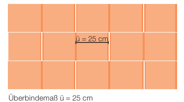
Verlegeschema Wandansicht
