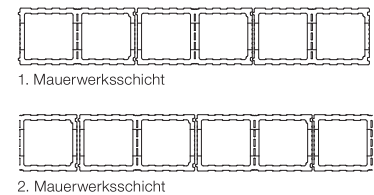
Verlegeschema Draufsicht
