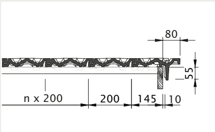
Ortgangausbildung mit Ortgangziegel rechts mit Ortgangbrett
