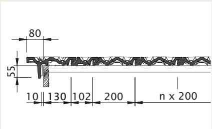
Ortgangausbildung mit Ortgangziegel links mit Ortgangbrett
