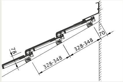
Wandanschluss (oben) mit Firstanschluss-Lüfterziegel
