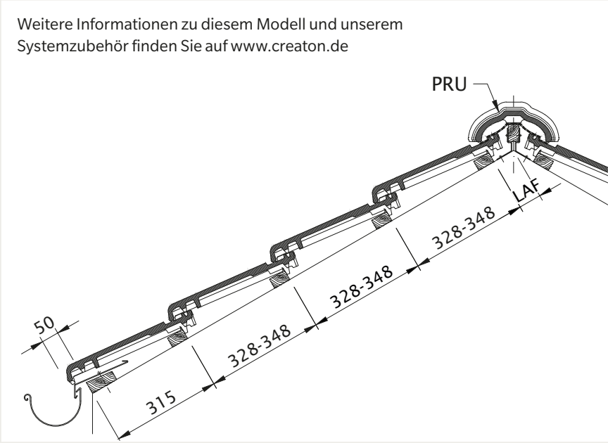
Dachquerschnitt Entlüftung über FALZ*. Firstziegel trocken verlegt. LQ bis ca. 230 cm²/m. First. Nach DIN 4108 bis 23 m Sparrenlänge. Traufplattenabstand variabel.
