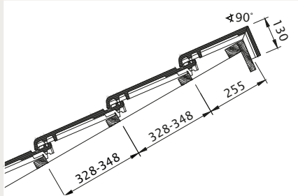
Pultdach-Ausführung
