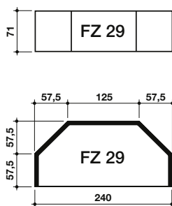
Breite 71 mm
