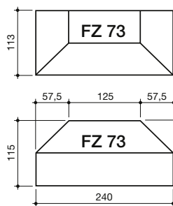
Breite 115 mm
