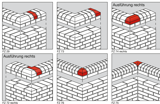
Breite 113 mm
