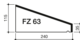
Breite 113 mm
